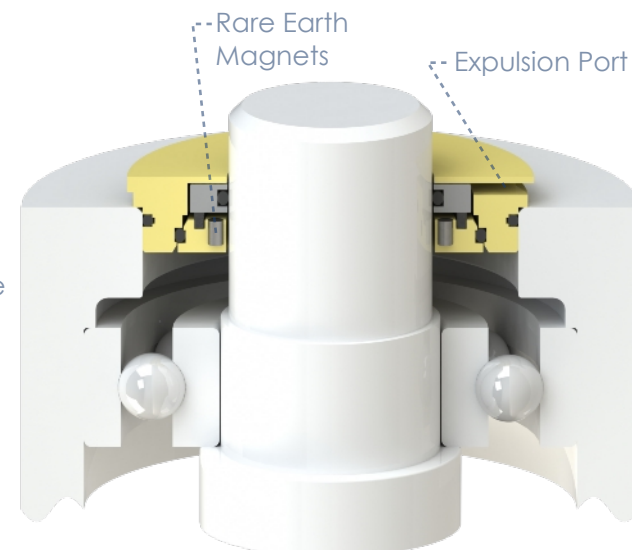
Magnum-D V8
